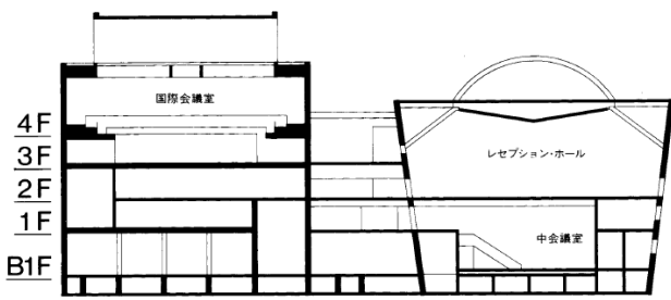
会議場棟断面図
